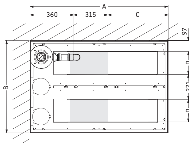
Posición de la conexión de desagüe
